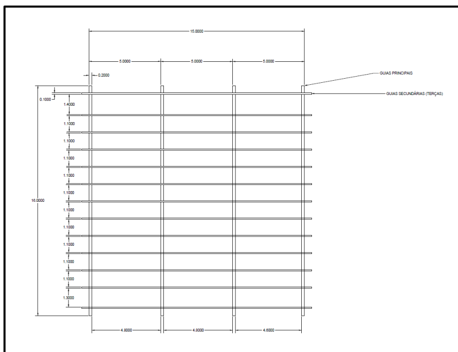
MALHA DE VIGAS PRIMÁRIAS E SECUNDÁRIA
