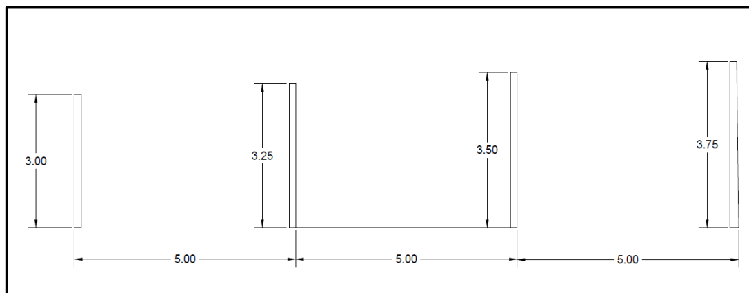
ARRANJO DE POSICIONAMENTO E ALTURA DOS PILARES
