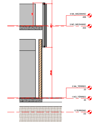
3 DETALHE GUARDA CORPO VARANDA ESCALA 1:20
