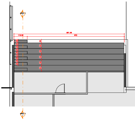
2. 2.NA TÉRREO - ARQUIBANCADAS ESCALA 1 : 50
