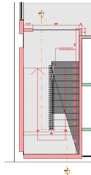
2 2.NA_TÉRREO - ESCADA ESCALA 1 : 25
