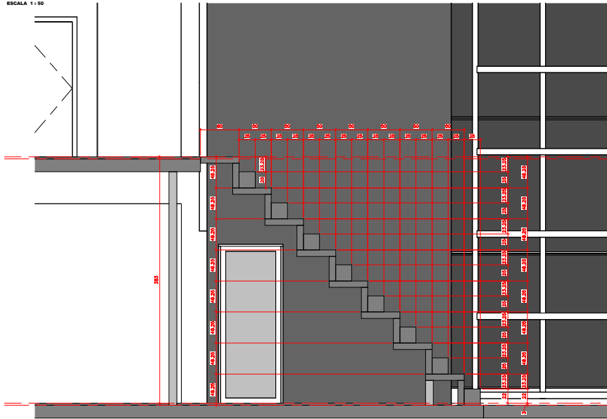
2. 2.NA TÉRREO - ARQUIBANCADAS ESCALA 1 : 50
