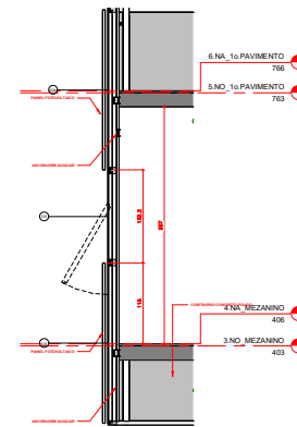
2 DETALHE GLAZING ESCALA 1:100
