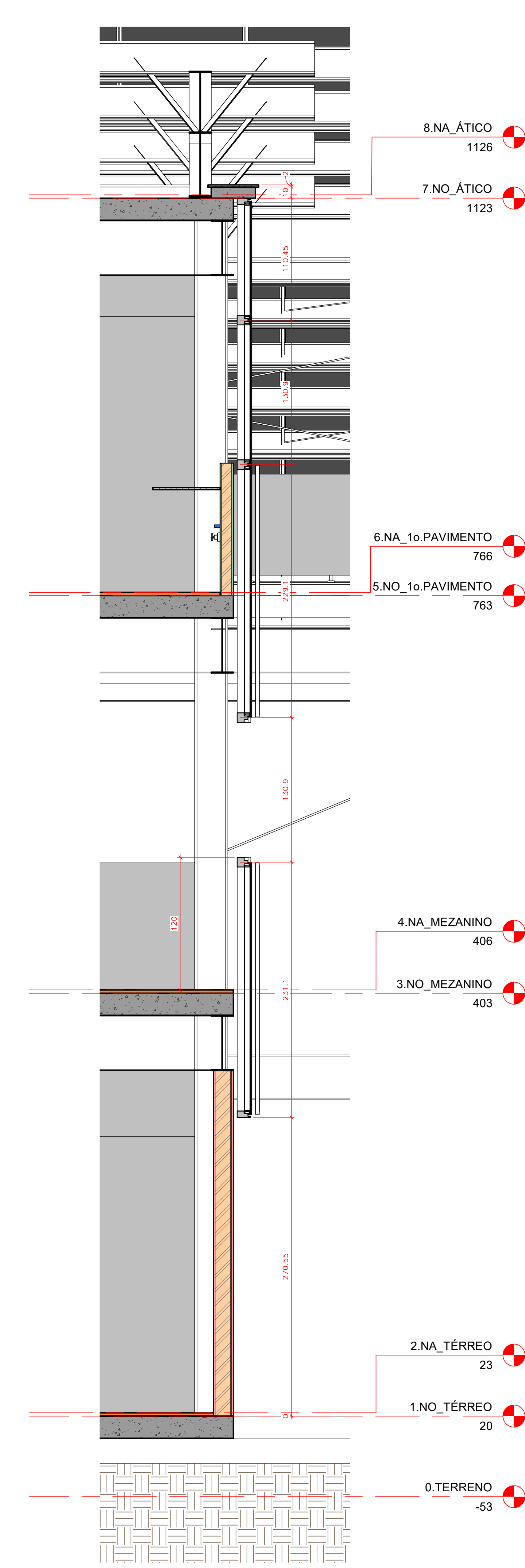
3 DETALHE GUARDA CORPO VARANDA ESCALA 1:25
