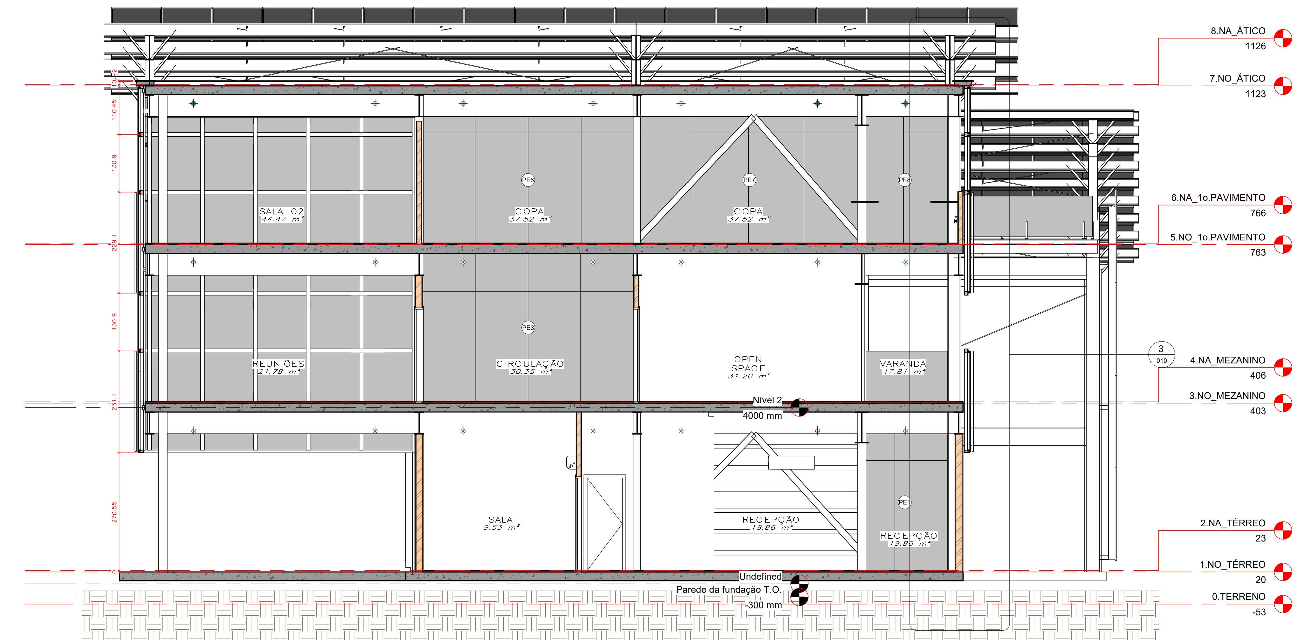
2 F ESCALA 1:50
