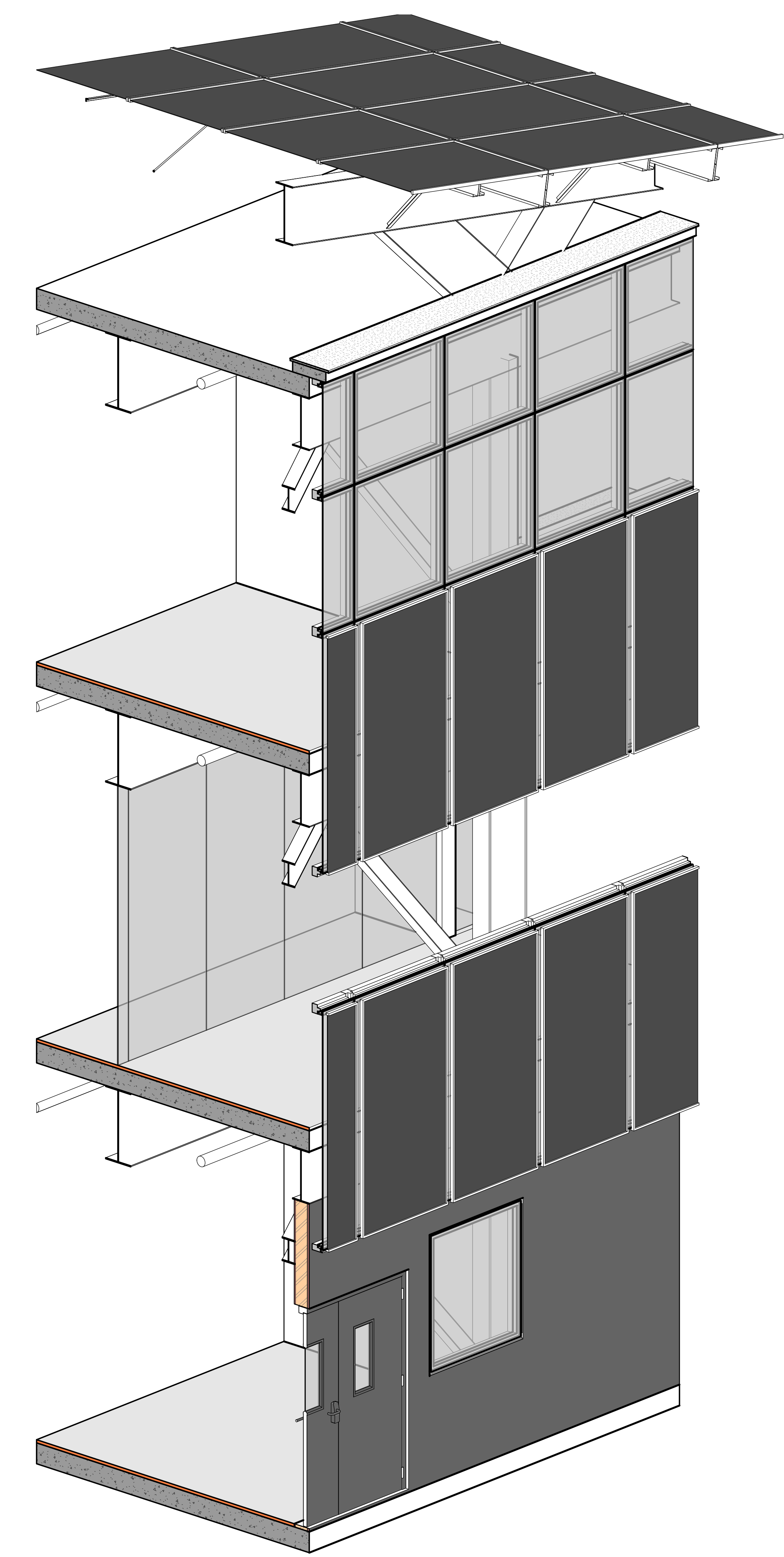
4 DETALHE GUARDA CORPO VARANDA ESCALA
